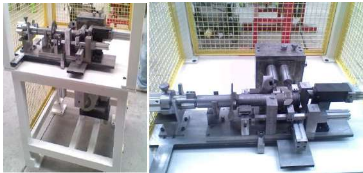
Desbarbadora
