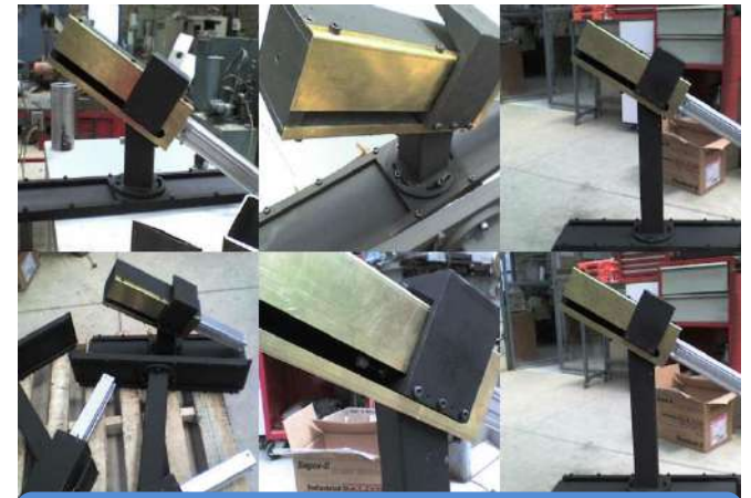
Estructura con pistón
