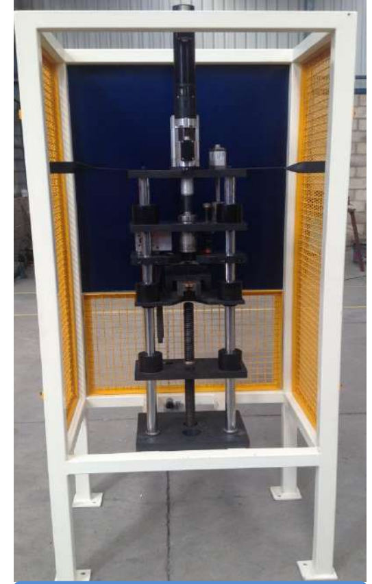
Prensa para roscar
