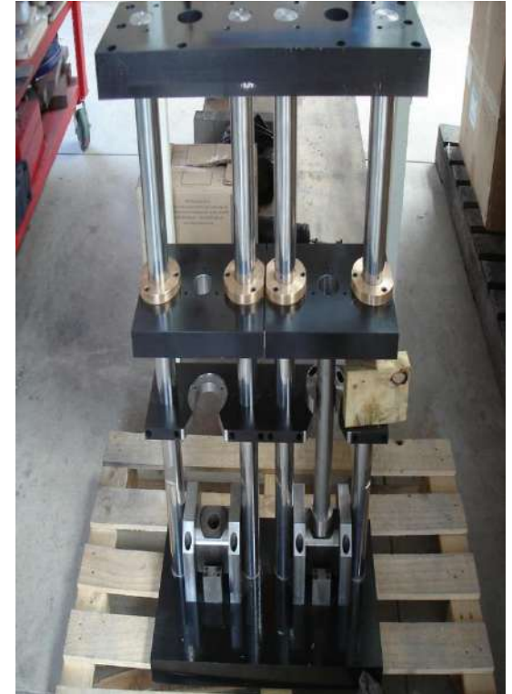
Prensa doble
